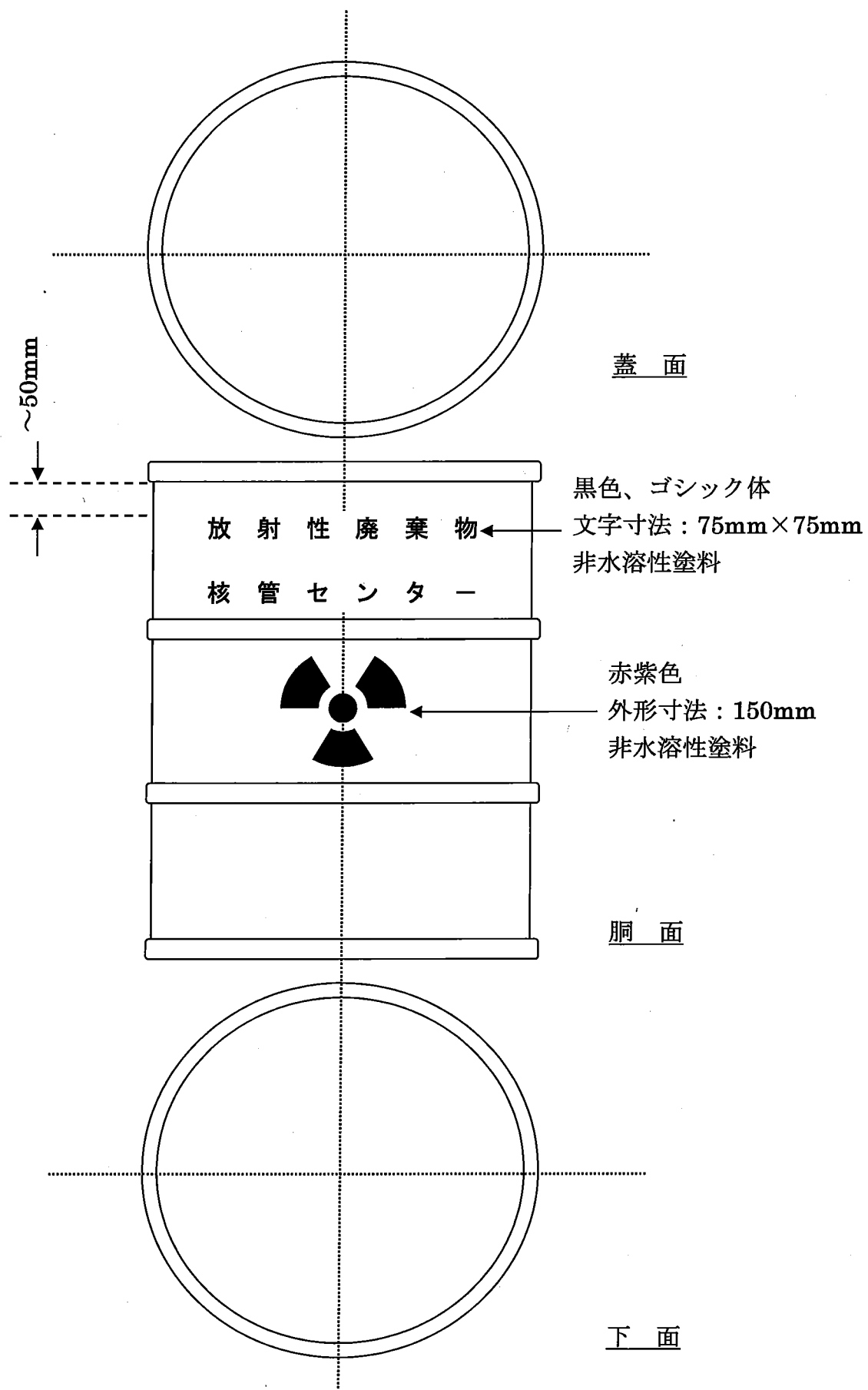
別添図 1 「文字、RI マークの印字」
